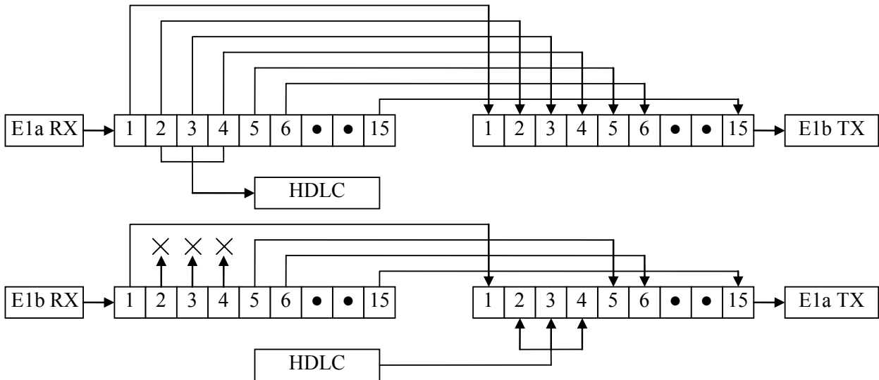
Рис. 10. Коммутация канальных интервалов в режиме drop-insert
