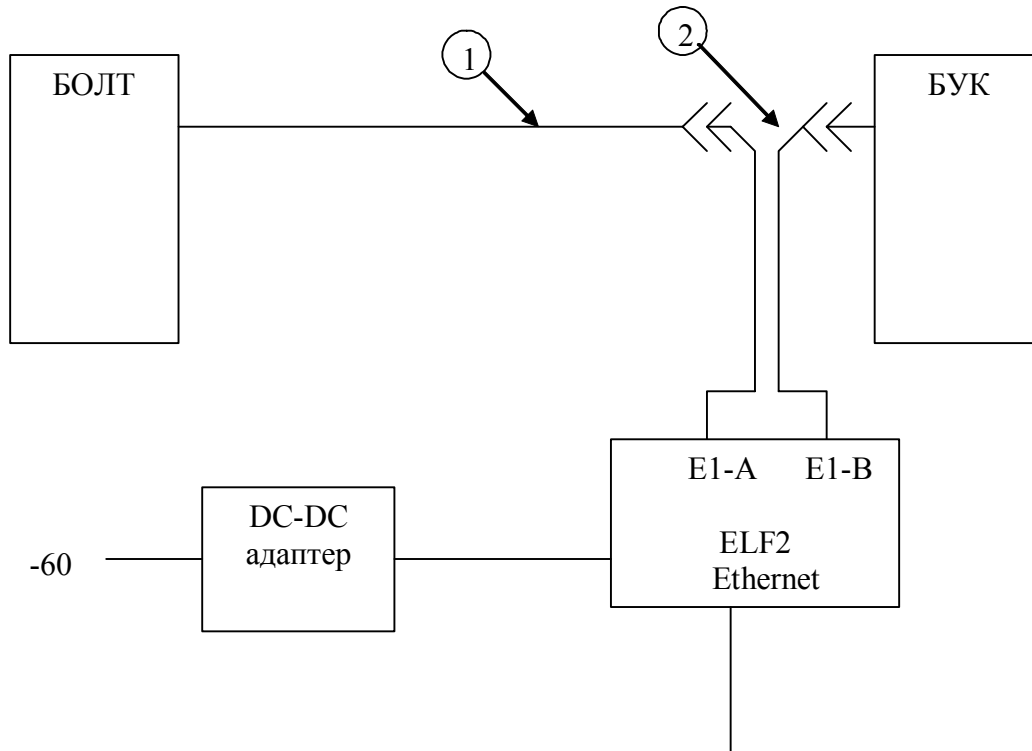
Рис. 2. Подключение к аппаратуре ИКМ-15
