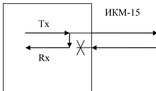
Рис. 6. Режим Lloop
