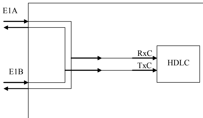
Рис. 11. Синхронизация в режиме drop-insert
