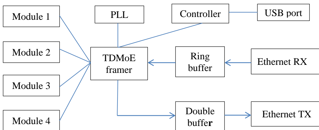
Рисунок 1. Блок-схема шасси Asteroid-1UT
