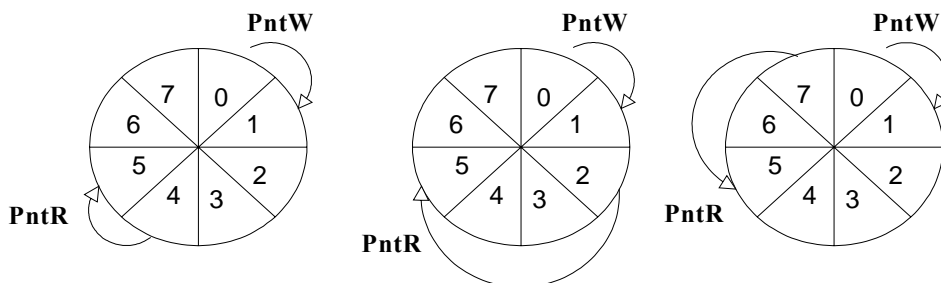
Рис. 3. Кольцевой буфер
