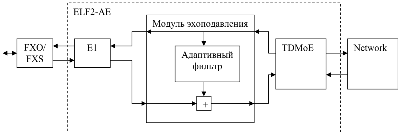
Рис. 10. Структура модуля эхоподавления
