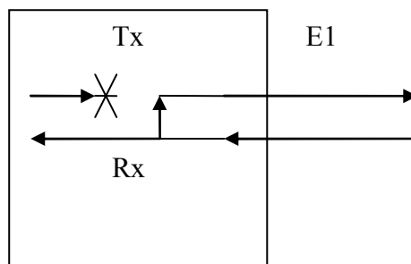
Рис. 8. Режим Rloop
